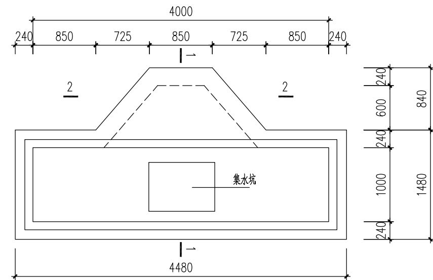
三通井平面示意图 1:50
