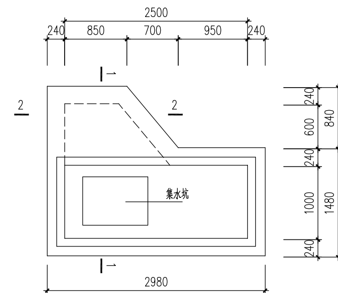
转角井平面示意图 1:50
