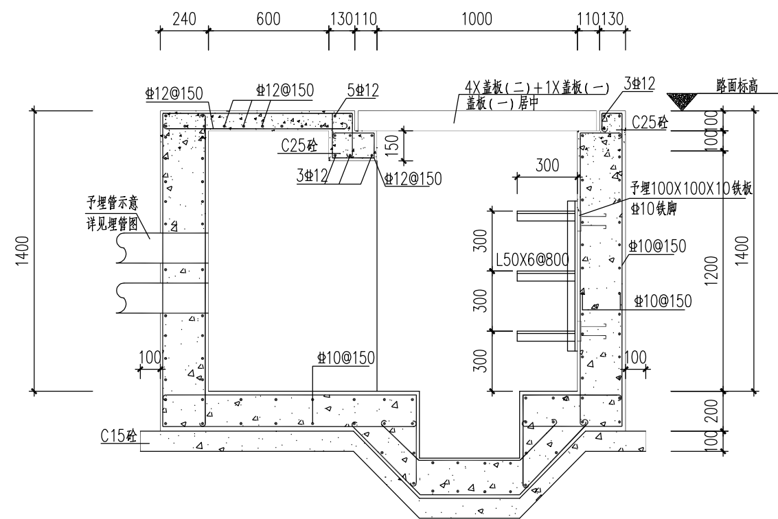
1-1剖面图 1:25
