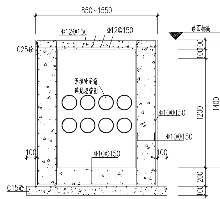
2-2剖面图 1:25
