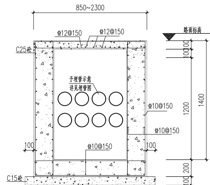
2-2剖面图 1:25
