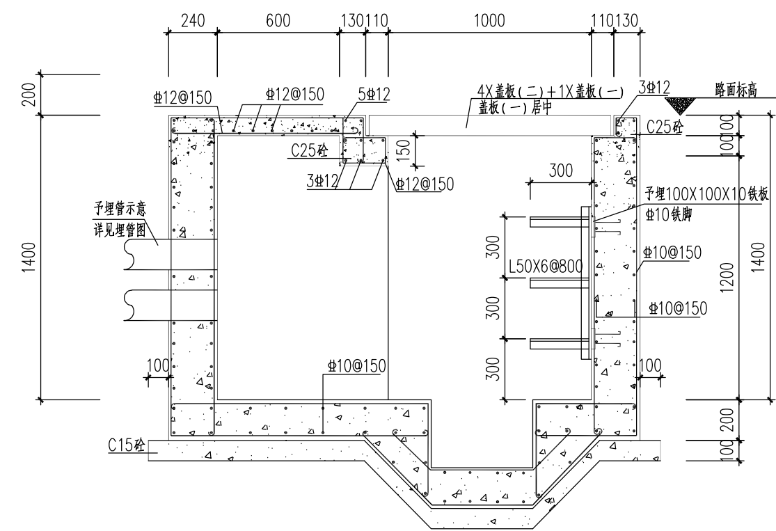
1-1剖面图 1:25
