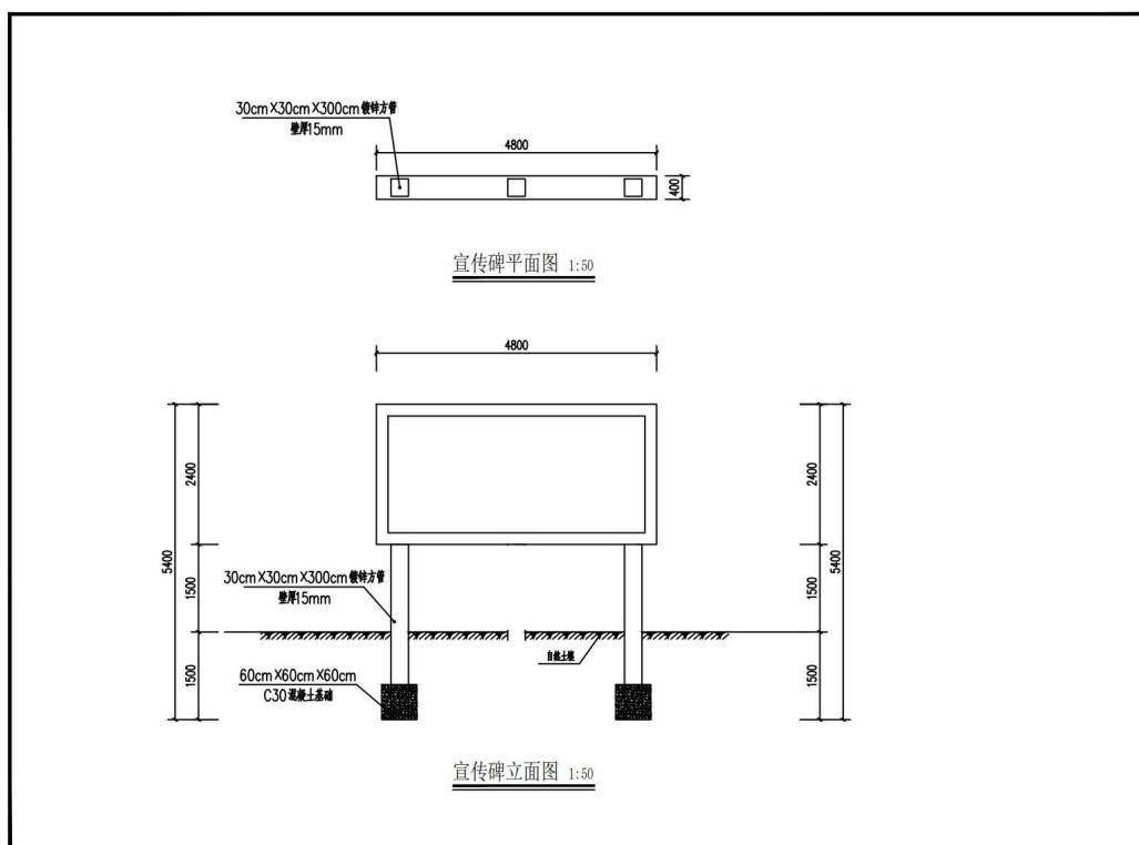
项目宣传碑设计图
