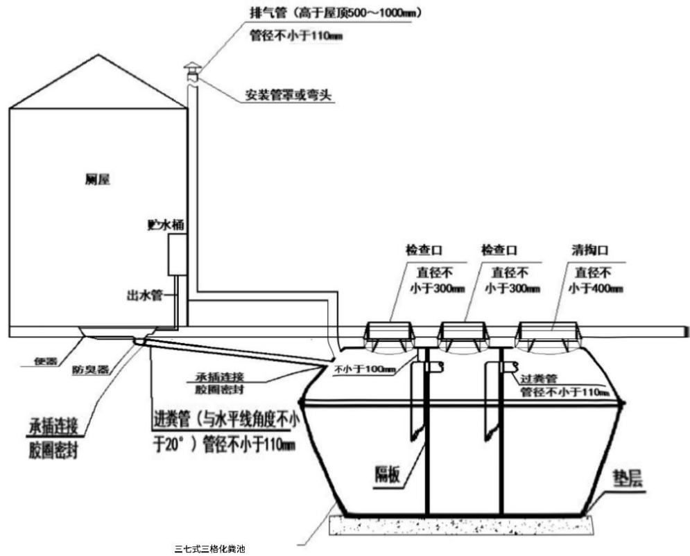
2、三七式三格化粪池管道连接图
