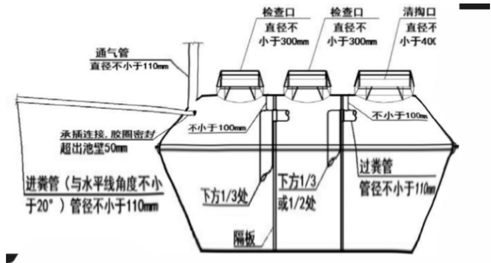
2、三七式三格化粪池管道连接图
